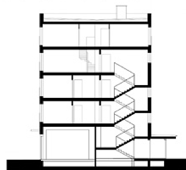
PRZEKRÓJ b-b
